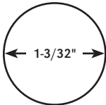
3/4" Conduit Knockout
